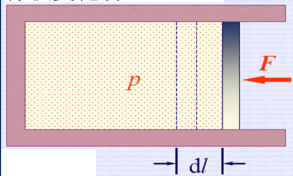
体积变化功
