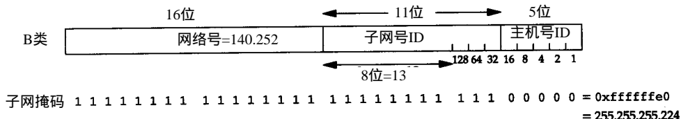
图3-11 变长子网
