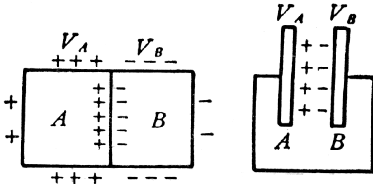
图 6-10 接触电势
