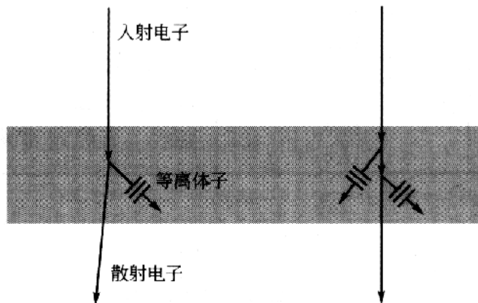
图6 在金属膜中借助电子的非弹性散射产生的等离体子。入射电子能量通常为 1~10eV ；等离体子能量数量级为10eV。图中还示出了产生两个等离体子的事例。
