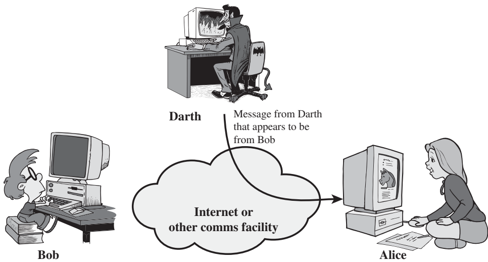
(a) Masquerade
