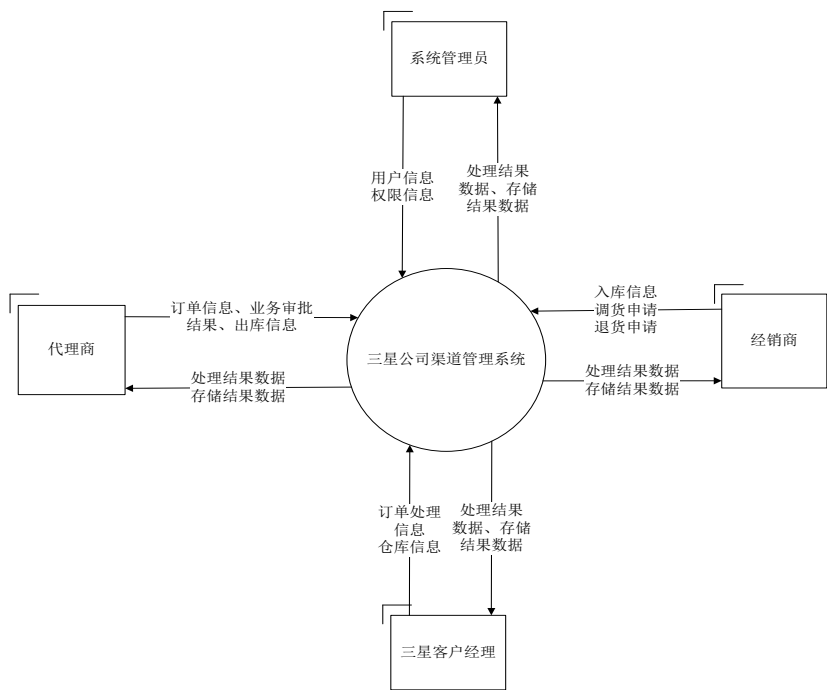
三星公司渠道管理系统的顶层数据流图
