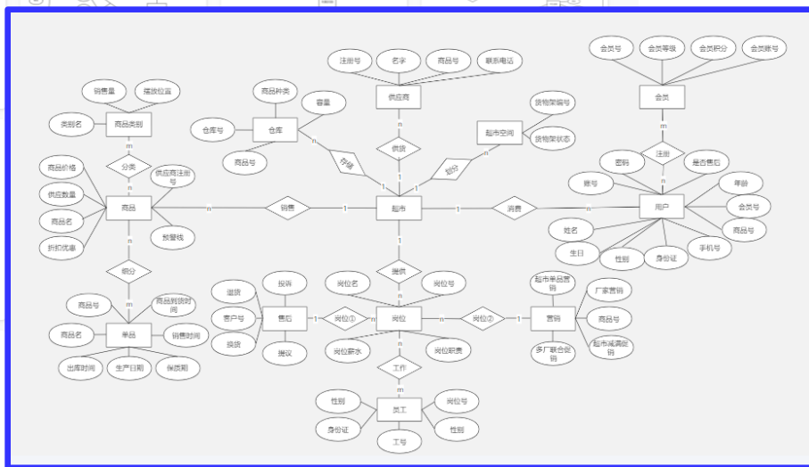
超市管理系统
