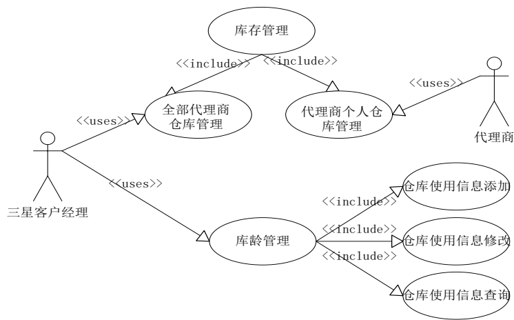
仓库管理需求用例图
