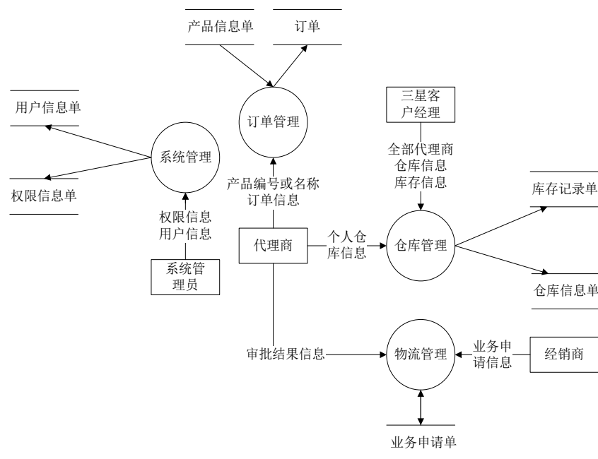
三星公司渠道管理系统1层数据流图
