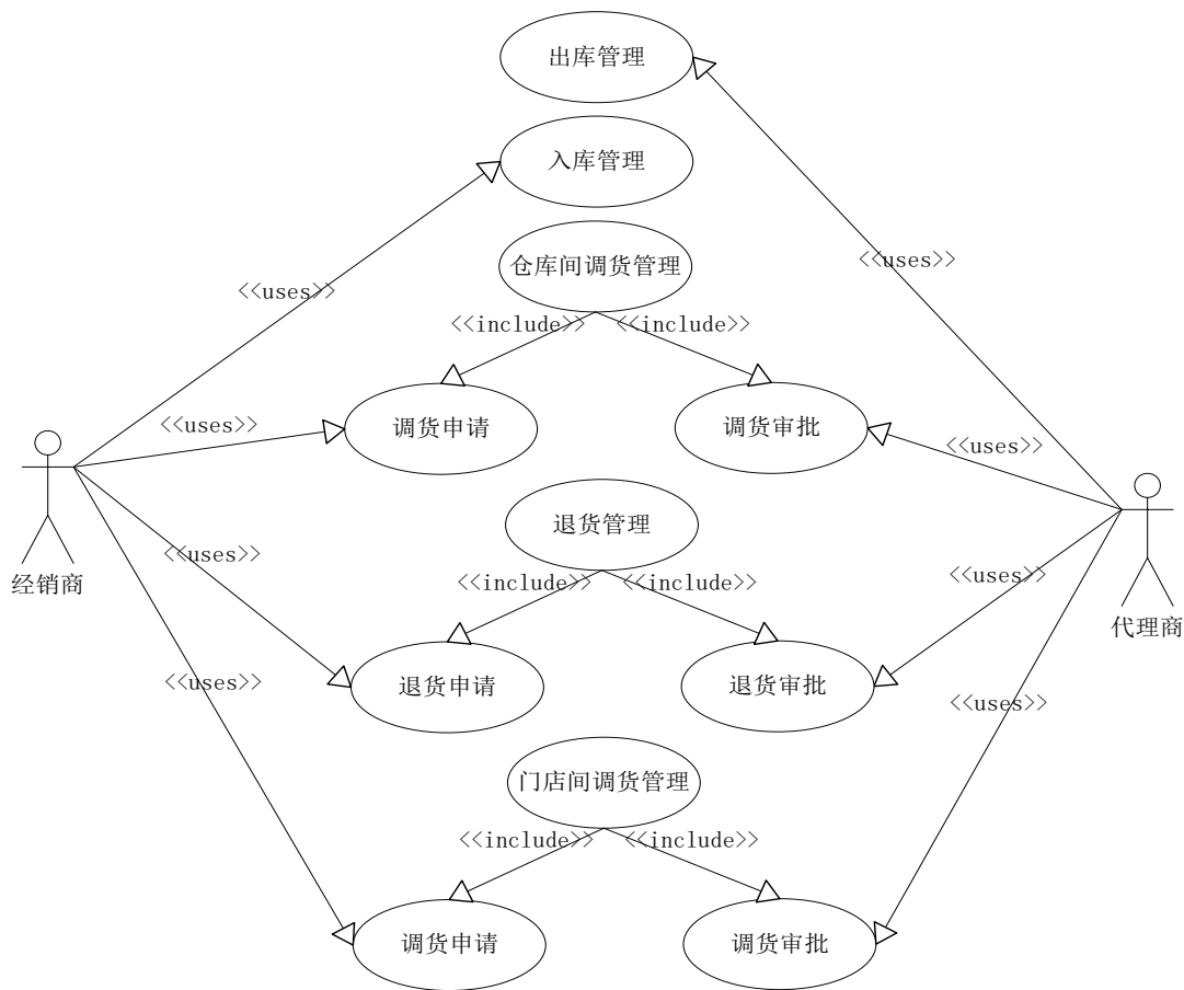
物流管理需求用例图
