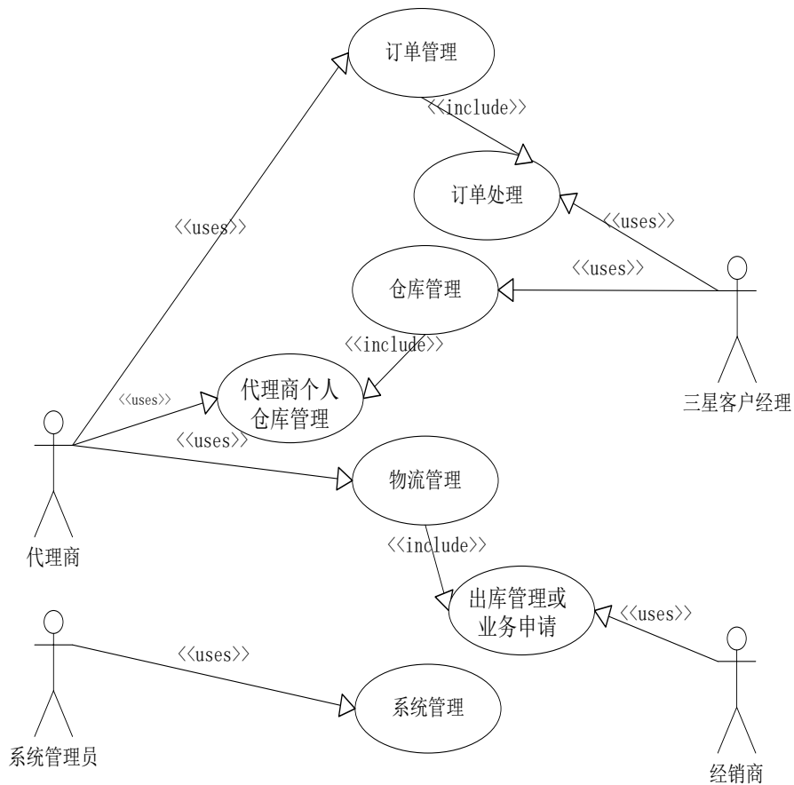
总体功能需求用例图
