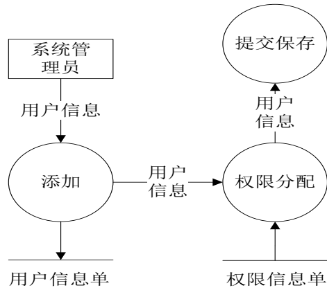
系统管理数据流图
