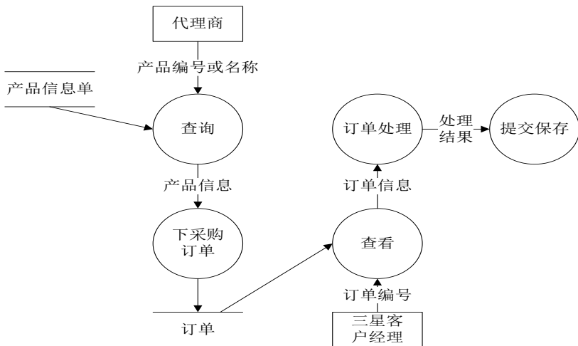
订单管理功能部分数据流图
