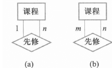
图7.8 单个实体型内的联系示例
