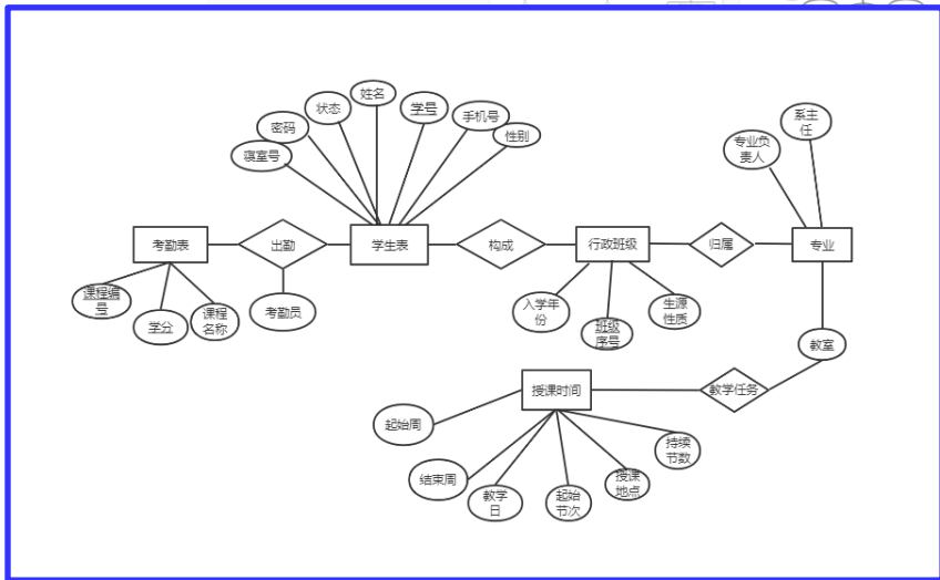
学生考勤管理系统
