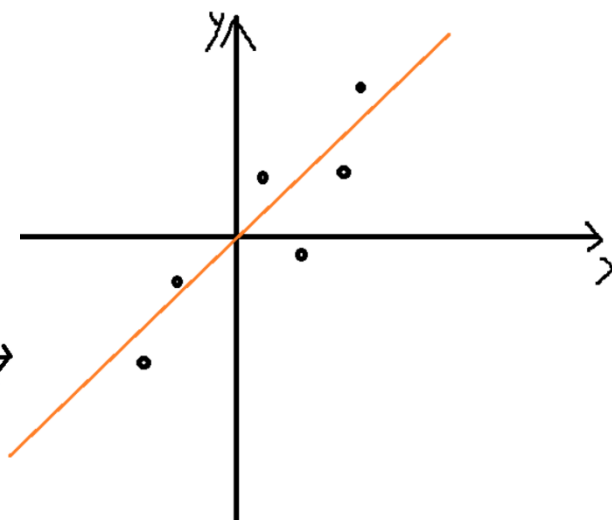
去中心化
