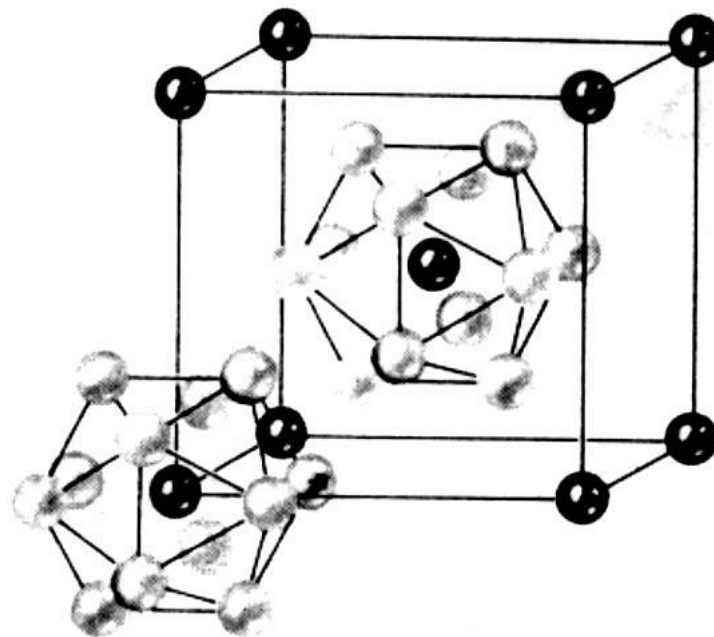
(b) MoAl 12 ; WAl 12 合金
