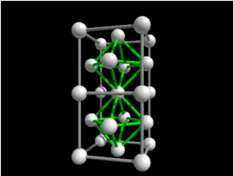
正八面体
