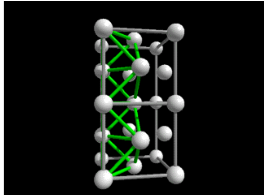
正四面体
