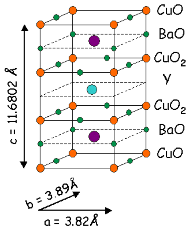
YBCO
