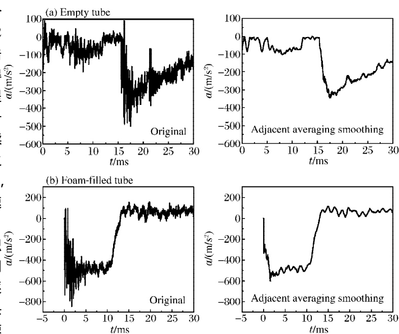
图2 典型落锤加速度-时间曲线
