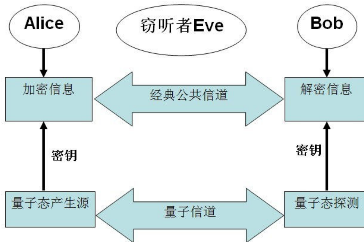
BB84协议示意图
