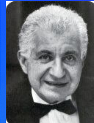
Boris Podolsky
