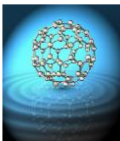
分子
