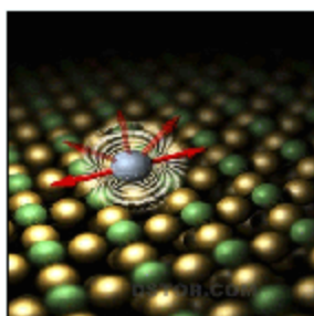
原子
