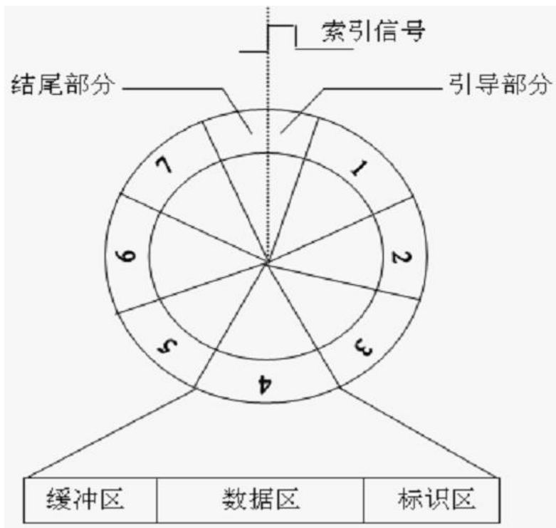
磁盘数据分布示意图
