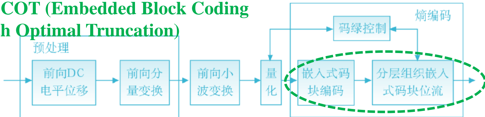
(a) JPEG2000编码器
