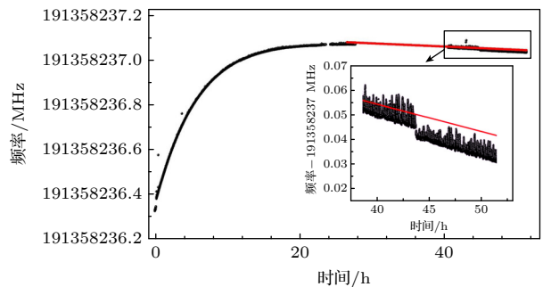
图 4 锁频激光频率随时间的变化
