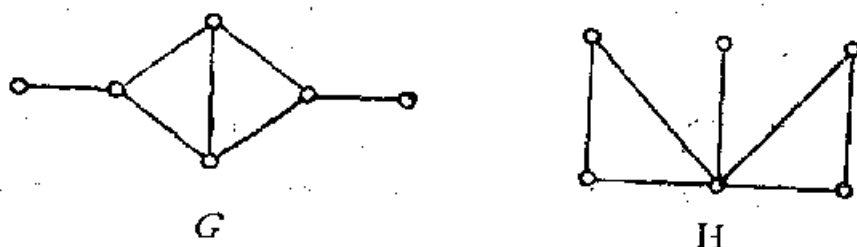
1.3.5 图
