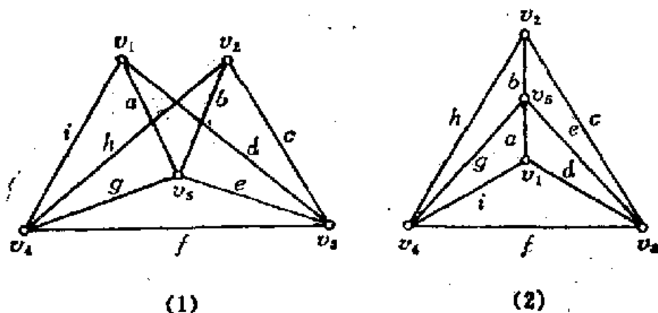
1.1.2 图
