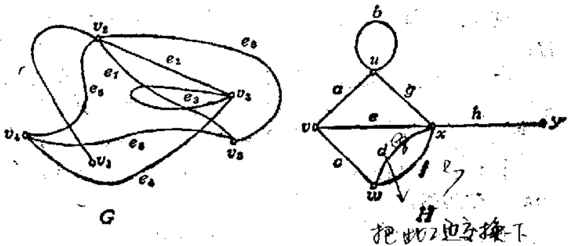
1.2.1 图
