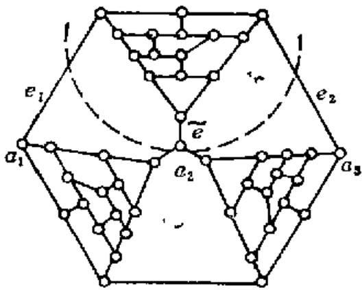
9-7.1 Tutte 图
