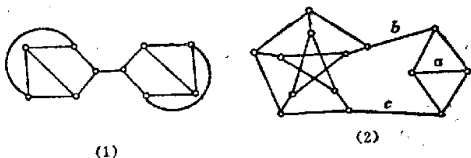
9.6.7 图
