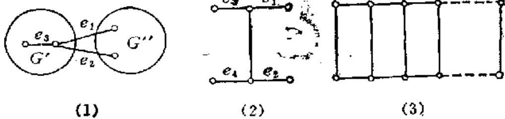
9.6.6 (a) 图
