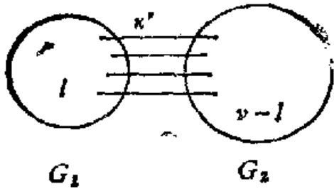
3.1.4 (a) 图
