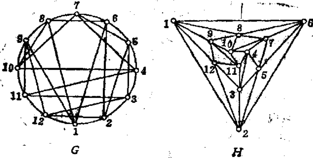
9.1.5 图
