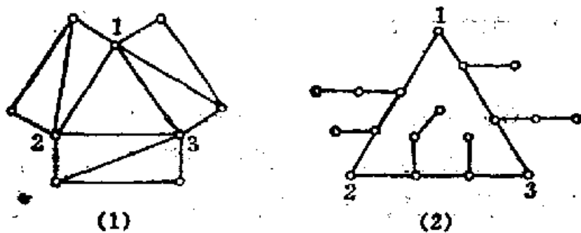
1.2.12 (f) 图
