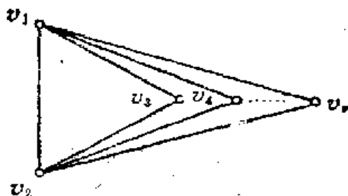
8.3.2 题图
