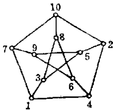
Petersen 图
