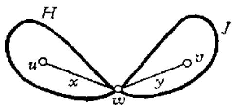
7.1.3 图
