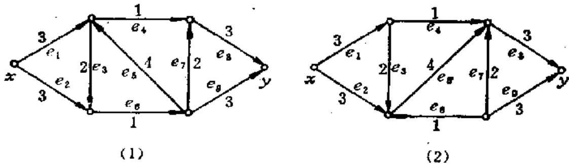
11.1.1 图
