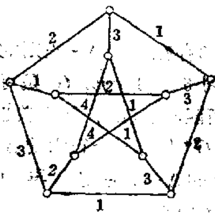
6.1.2图
