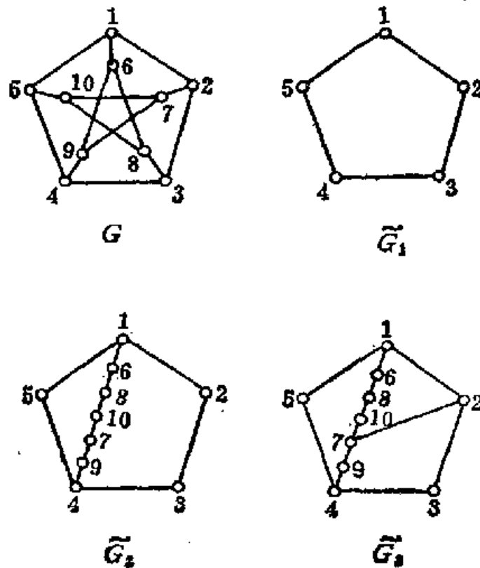
9.8.1 图
