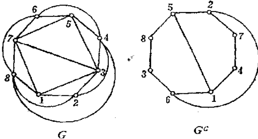
9.3.3 (b) 图
