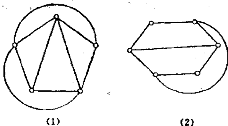
9.1.2 图
