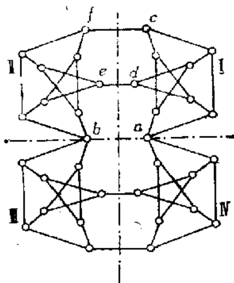
Thomassen 图
