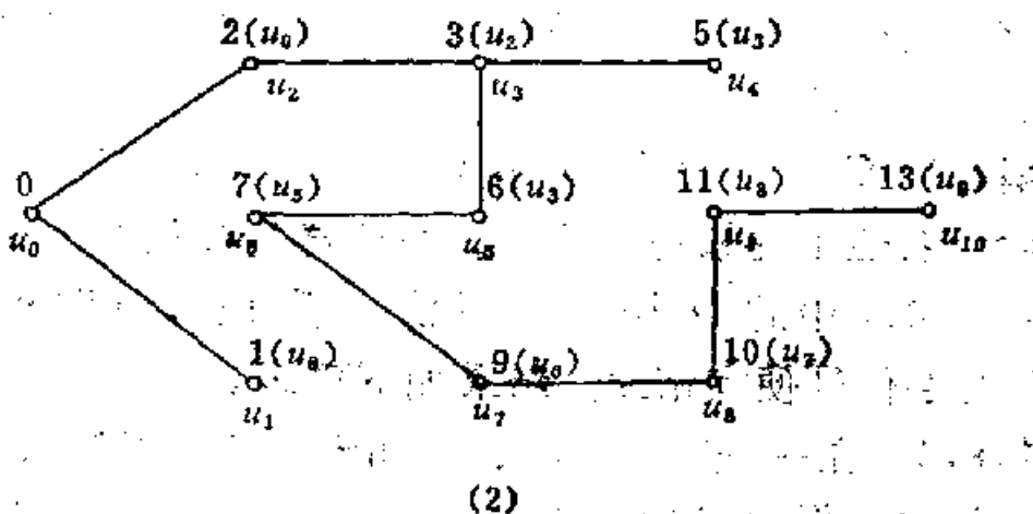
1.8.1 图
