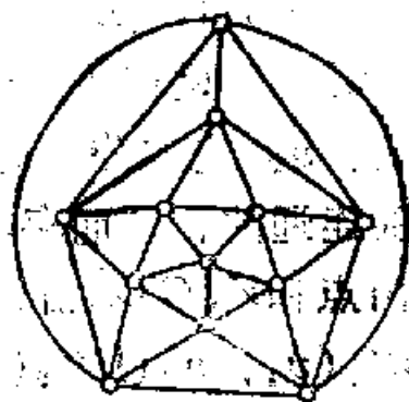
9.3.9(b)图
