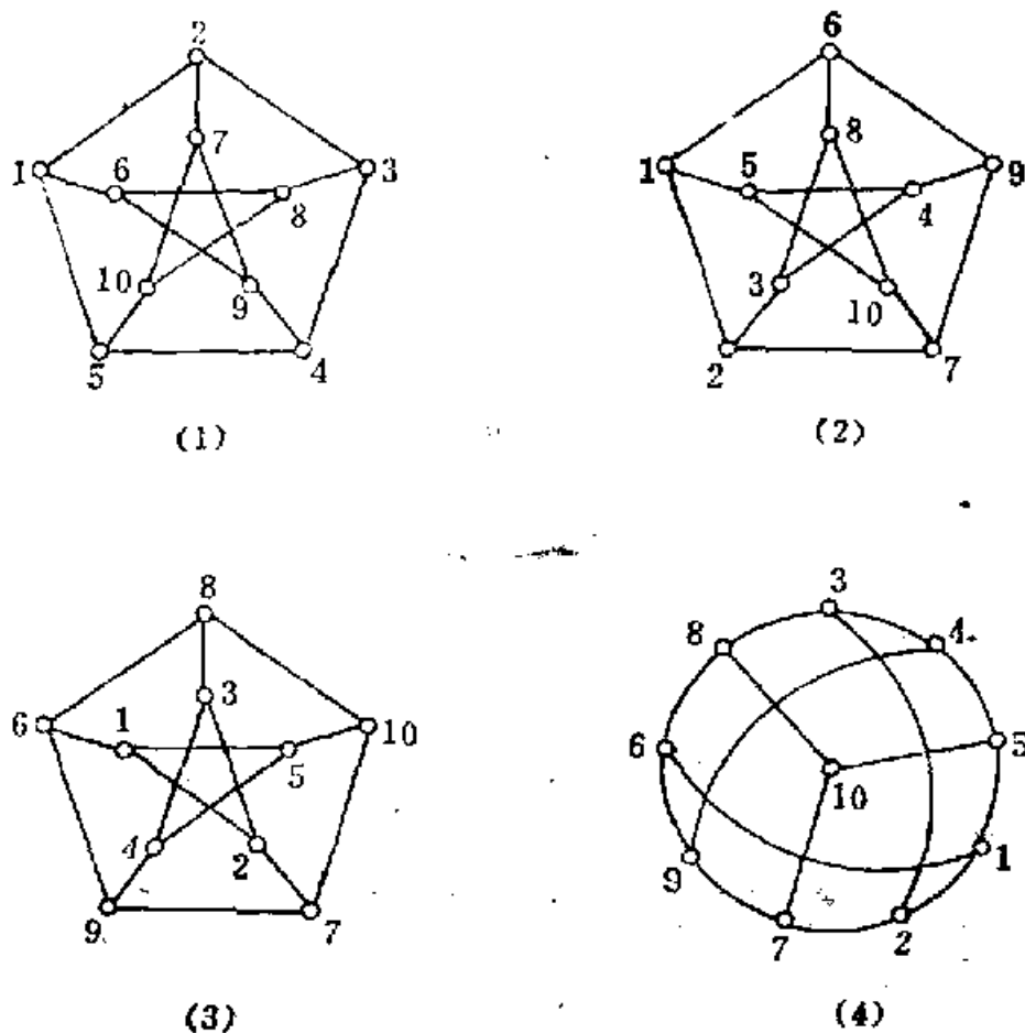
4.2.12 图
