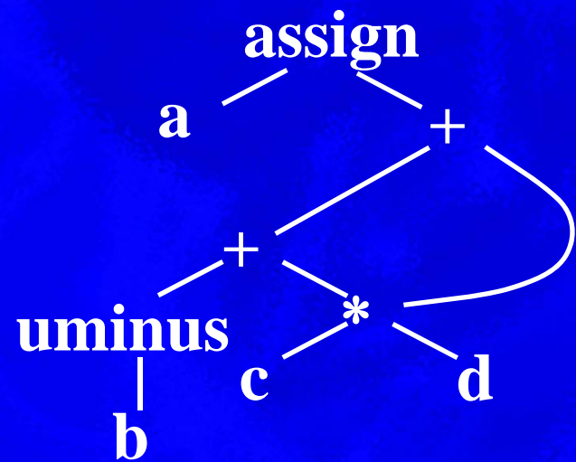
(b) DAG
