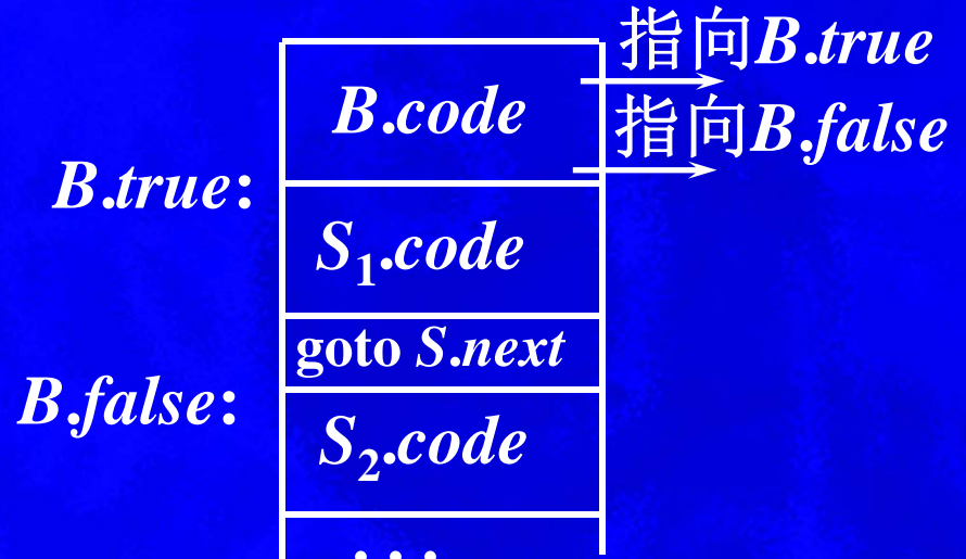
(b) if-then-else
