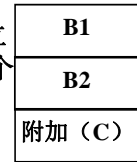
独立的多重继承时的对象结构 (程序视图)
