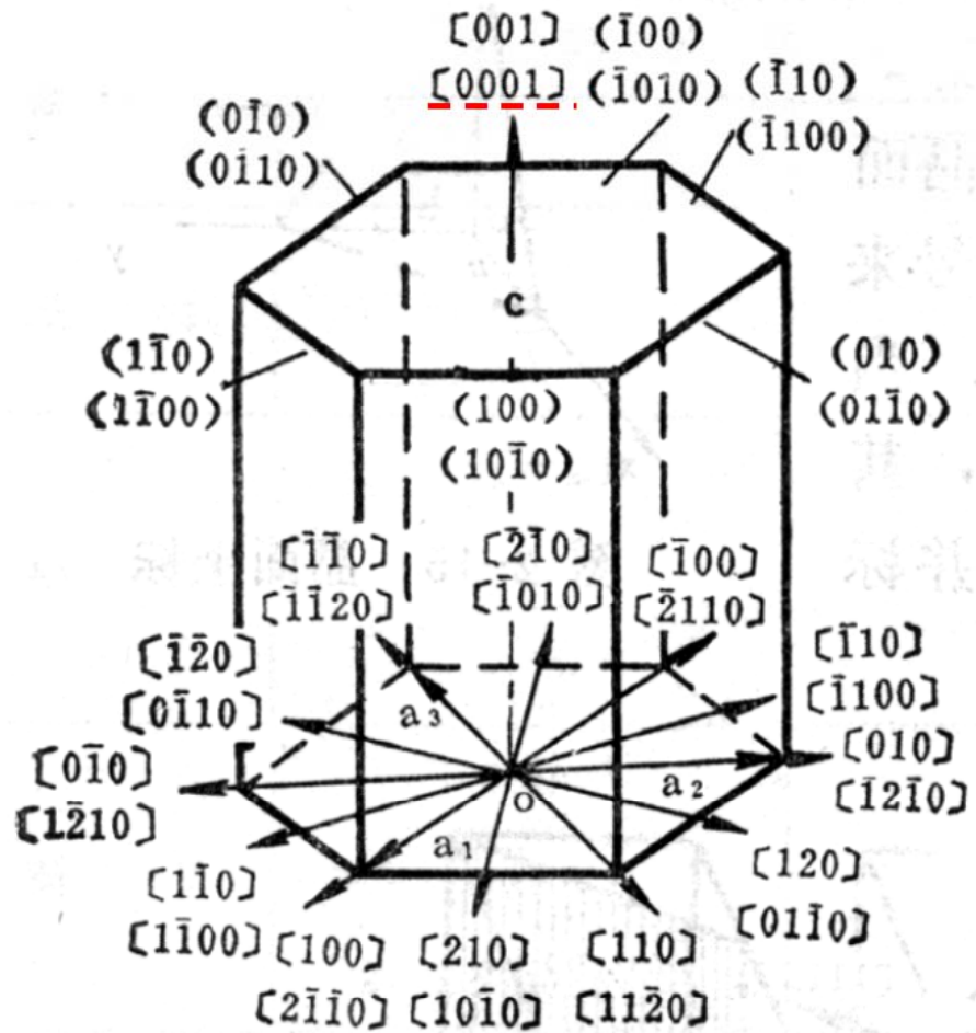
六方晶系的晶面及晶向指数
