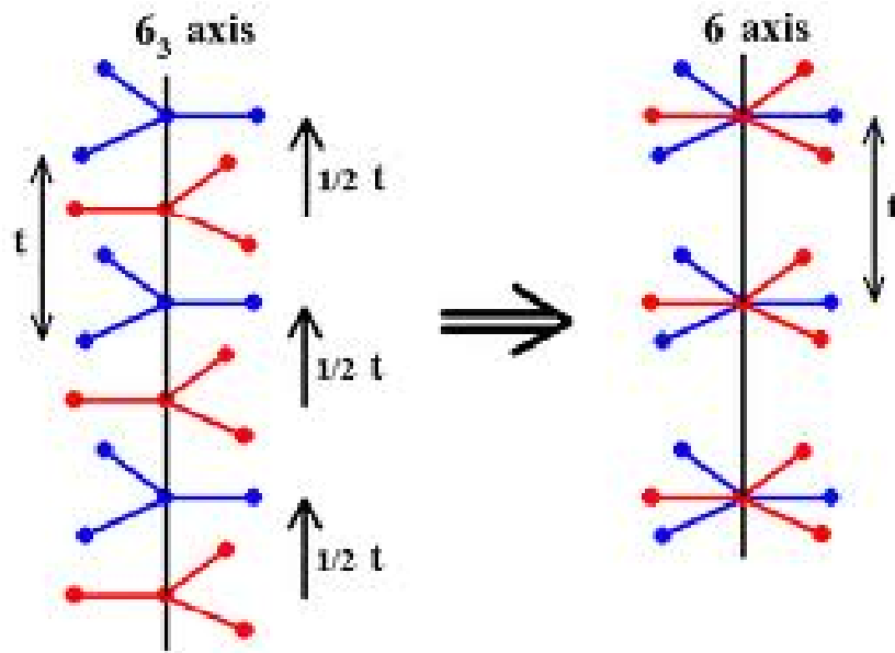
6度螺旋轴 (screw axis) n 度螺旋轴是旋转 2\pi/n 与 沿轴向平移的复合操作
