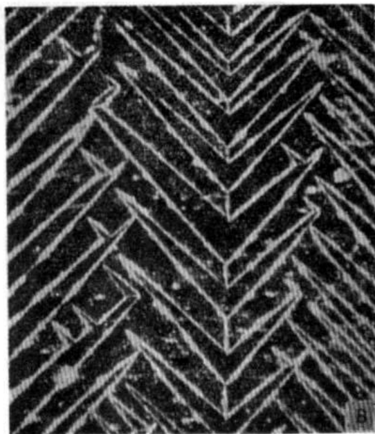
(b) 在同一表面上经过电解抛光后的粉纹图型.
