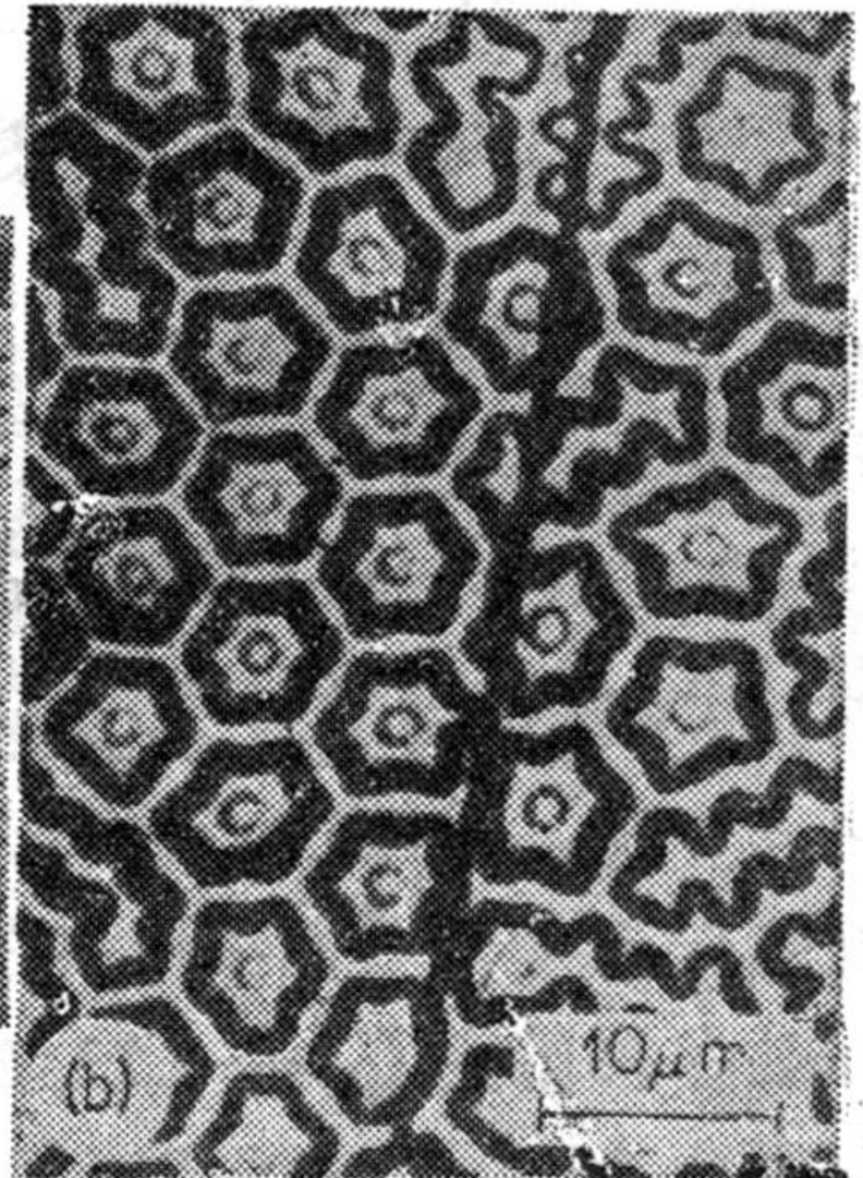
图 8.20 Ba 铁氧体单晶基面上的磁畴图形。
