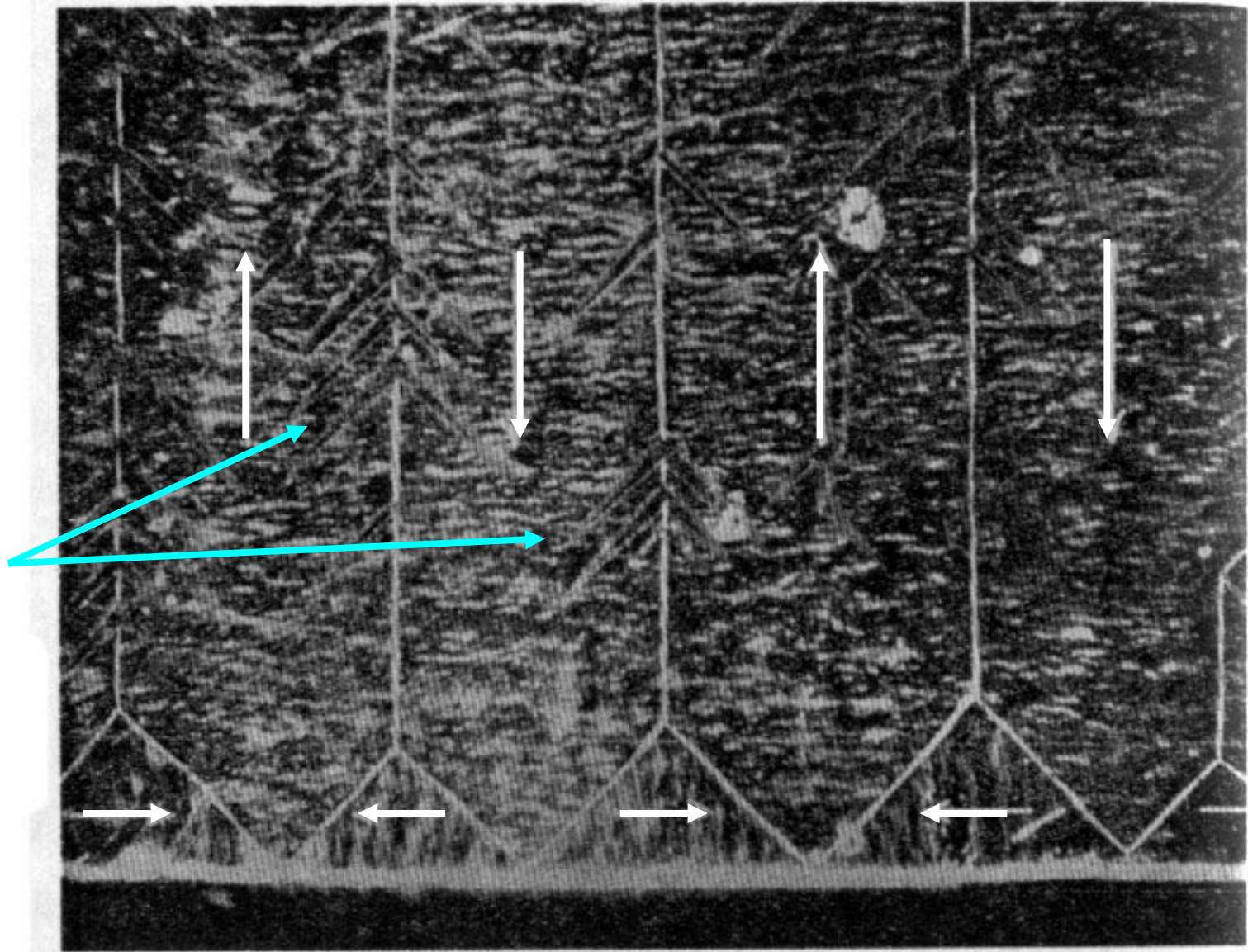
硅鉄晶体 (100) 表面的粉紋图型。 晶軸 +
