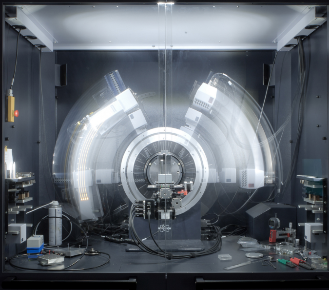
图 - 运行中的粉末 X 射线衍射仪 (图源wikipedia)
