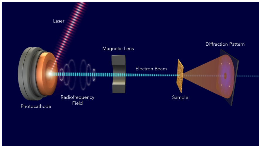
图 - 超快电子衍射实验设备示意图 16
