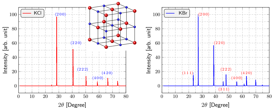
图 - KCl (左) 和 KBr (右) 的粉末样品 X 射线衍射谱。
